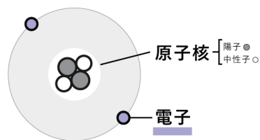
原子模式図
